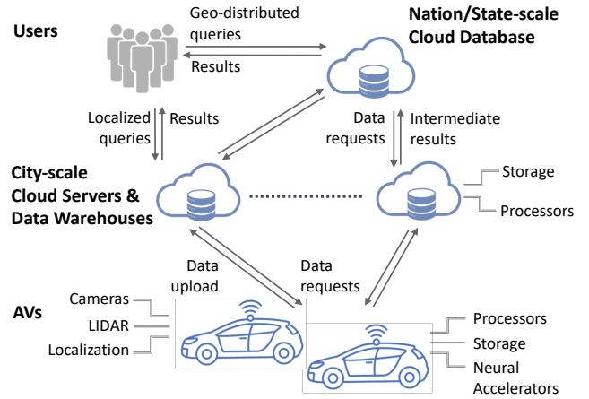
Figure 2: AV query system architecture
